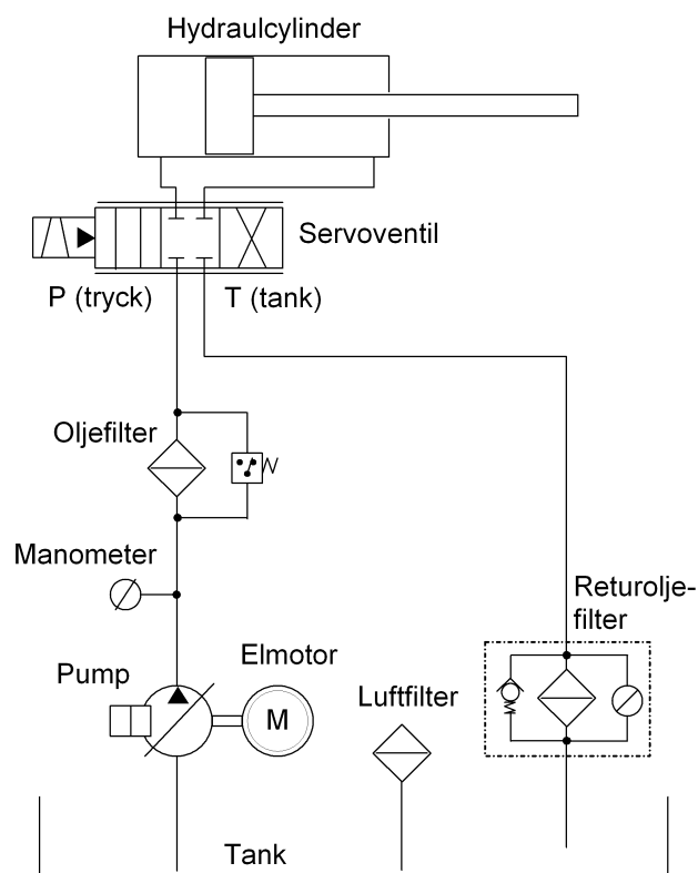
Figur 7.2 Exempel på hydraulsystem.
