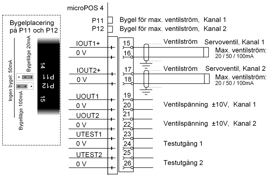
Figur 3.6 Anslutning av servoventiler, och byglar för strömmråde. Testutgångarna är avsedda för mätning.
