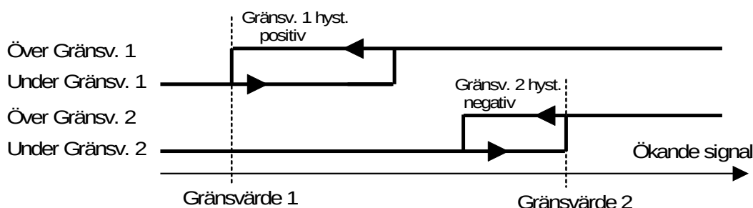
Figur 13. Hysteresens inverkan på nivåövervakningen.
