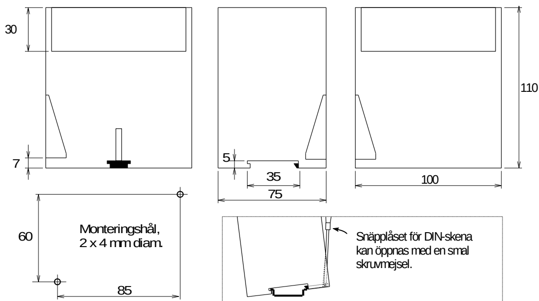
Figur 3. Mekaniska dimensioner för AST 3.
